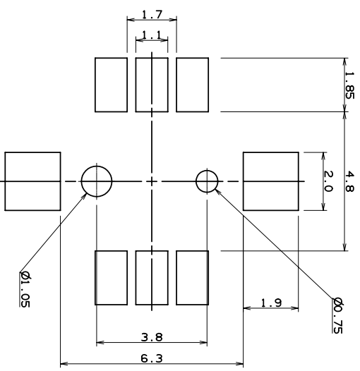
P.C.B DIMENSION
